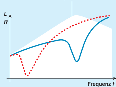
Bild 15 Schalltechnische Auslegung von KS-Außenwänden mit WDV in Abhängigkeit vom vorliegenden Außenlärmspektrum
